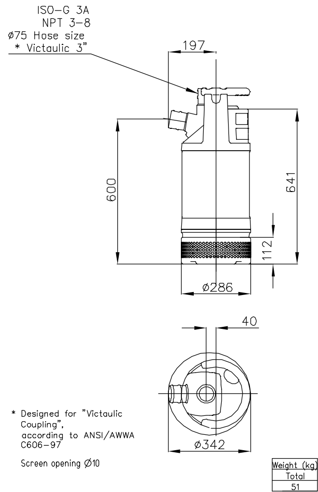
Figura 12: BS/KS, versão padrão, HT
