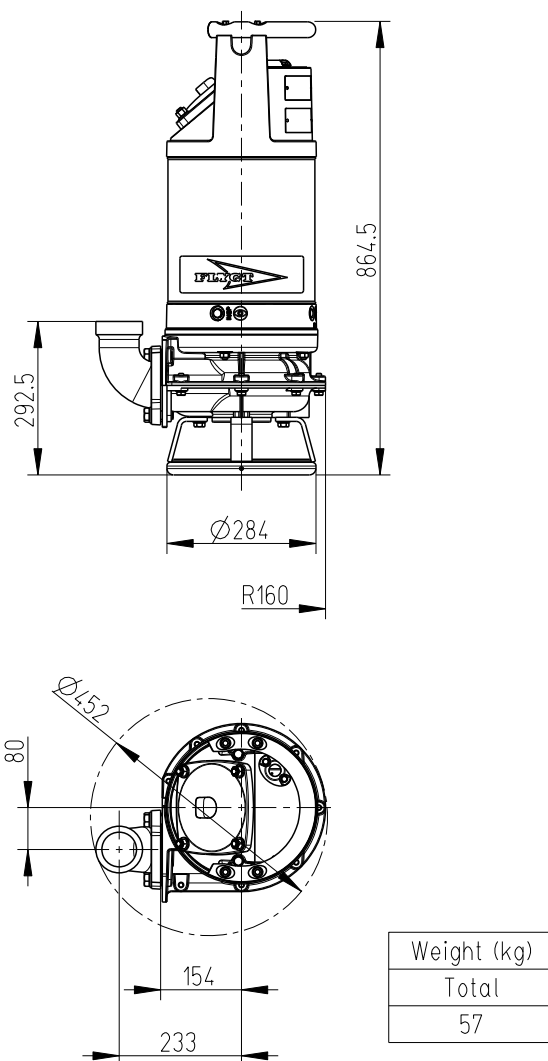
Figura 13: DS, versão padrão
