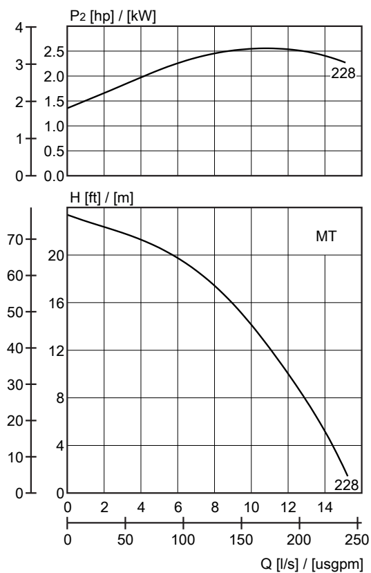
Figura 18: BS, trifásico
