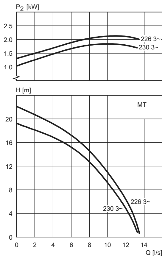
Figura 12: BS, trifásico
