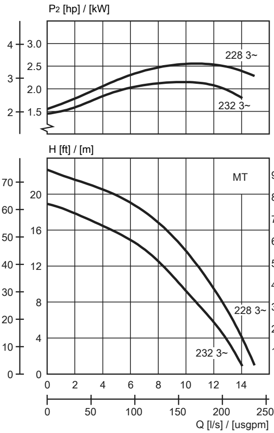
Figura 15: BS, trifásico
