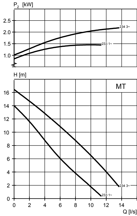
Figura 14: Monofásico, trifásico
