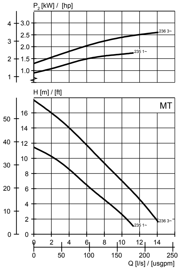
Figura 17: Monofásico, trifásico
