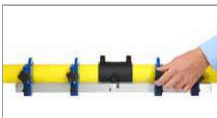
8. Utilizar um posicionador para fixar o tubo.
